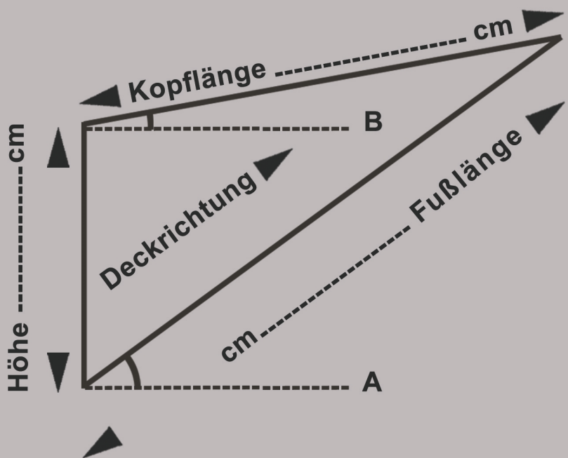
rechte Gaubenwange
